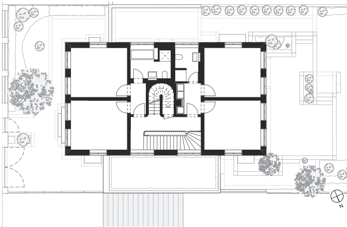
05 Grundriss Obergeschoss
