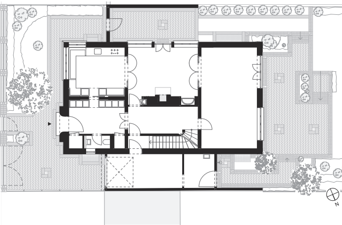
04 Grundriss Erdgeschoss
